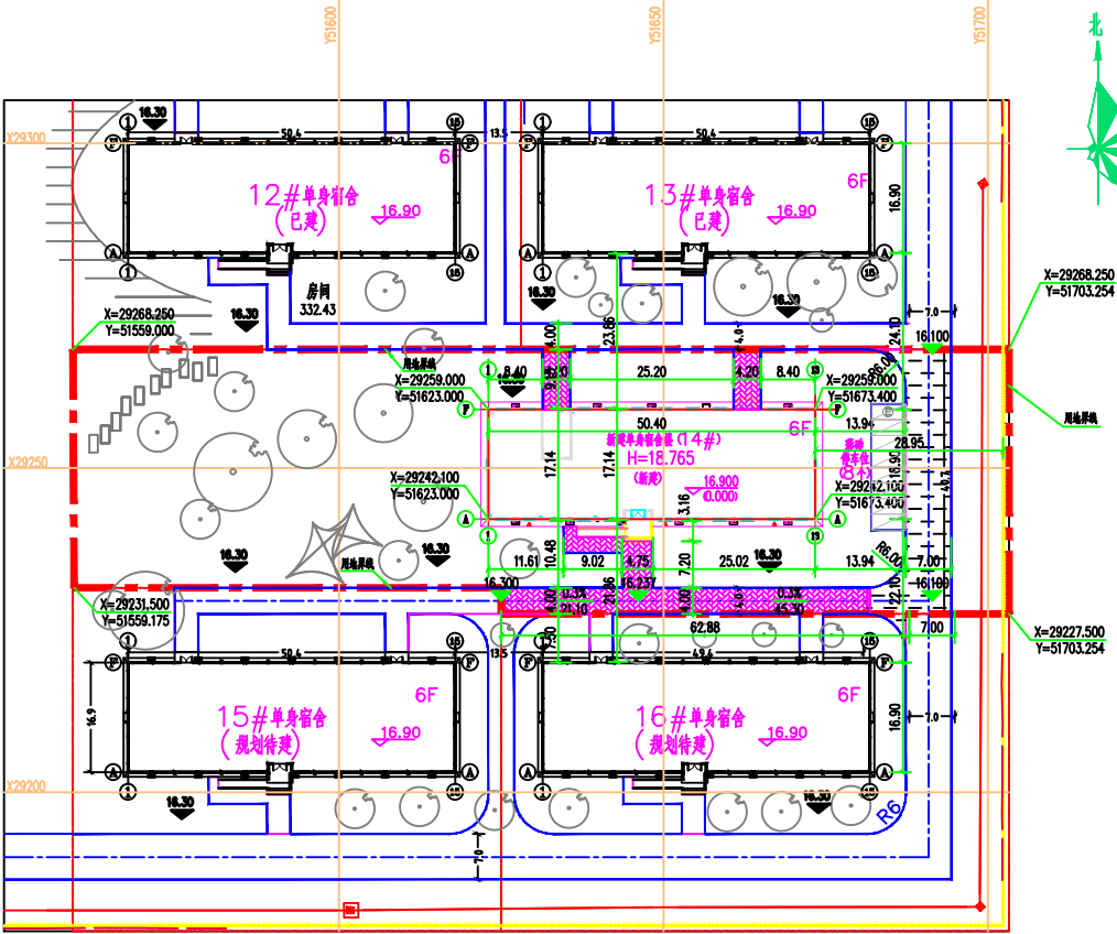
总平面布置图 1:500
